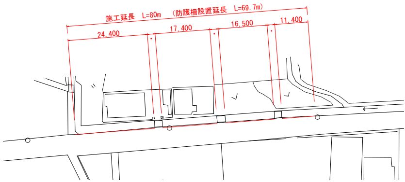
転落防止柵 S=1:20
